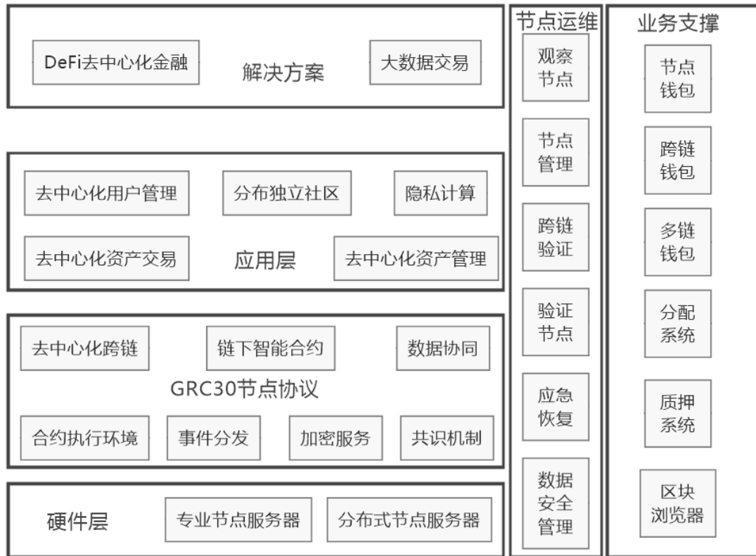
图 1 银河公链技术架构图
